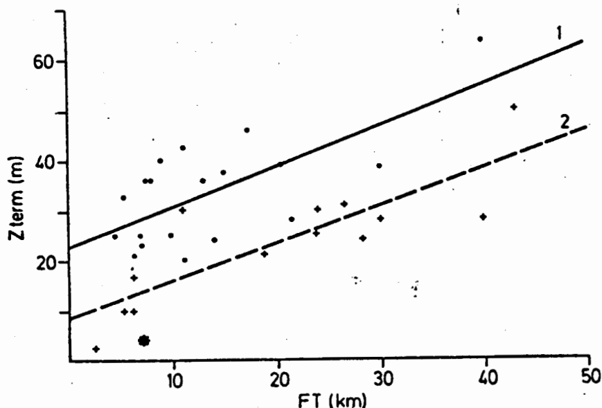
Fig. 2. Relación entre la profundidad de la termoclina a fines del verano ( Z_{term} ) y el alcance del viento (FT). • Lagos y embalses argentinos (recta 1); + lagos chilenos (recta 2); * Laguna Blanca (Argentina).
