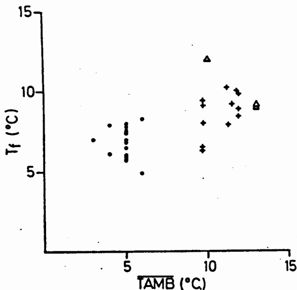
Fig. 7. Agrupamiento de los ambientes lacustres de la Región Andino-Patagónica según la temperatura media anual del ambiente ( T_{AMB} ) y la temperatura de las aguas profundas ( T_f ). • lagos argentinos; + lagos chilenos; \triangle lagos y embalses de la meseta patagónica.
