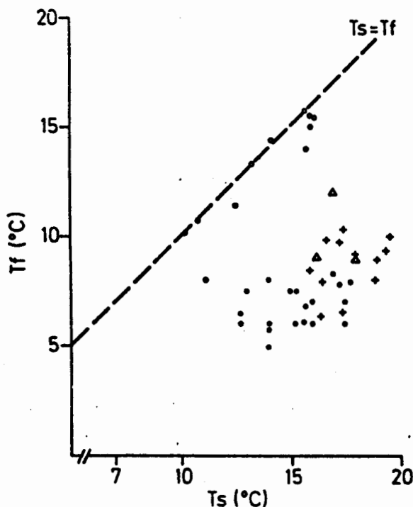
Fig. 6. Temperatura de las aguas superficiales ( T_s ) y profundas ( T_f ) en ambientes lacustres de la Región Andino-Patagónica. • Lagos argentinos; + lagos chilenos; \Delta lagos y embalses de la meseta patagónica; \circ lagos no estratificados.
