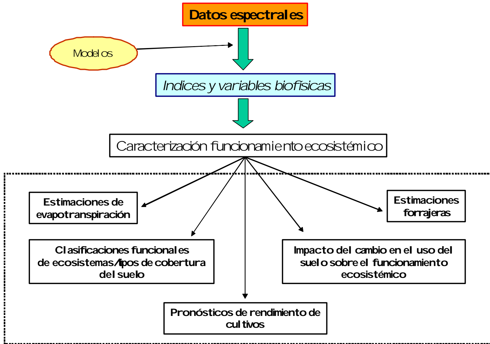
Figura 3. Esquema de generación de aplicaciones de la teledetección a partir de la traducción de los datos espectrales en variables biofísicas y en la caracterización del funcionamiento ecosistémico a partir de ellas.
